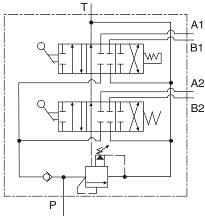
ZS1-L10※-OT.OW
