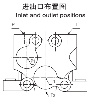
压力分级及进回油口位置/PRESSURE GRADE、INLET AND OUTLET POSITIONS 表1/Table 1
