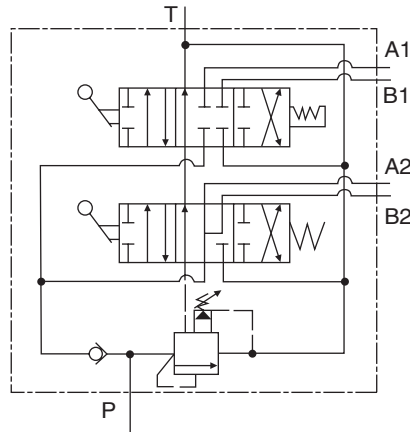
ZS1-L10※-YT.OW
