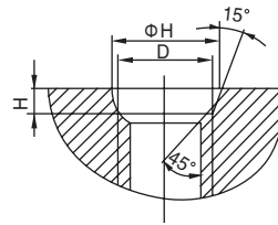
油口尺寸
