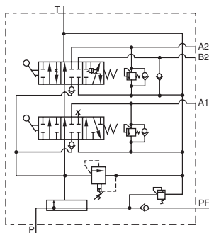
CDB-F15-A5T.R3T
